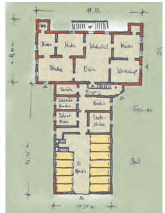
Abbildungen auf dieser Seite: Der Architekt Manfred Blanke hat zeichnerisch rekonstruiert, wie die Gebäude früher ausgesehen haben könnten. oben: das Hallenhaus, Mitte: Grundriss frühes 19. Jahrhundert
